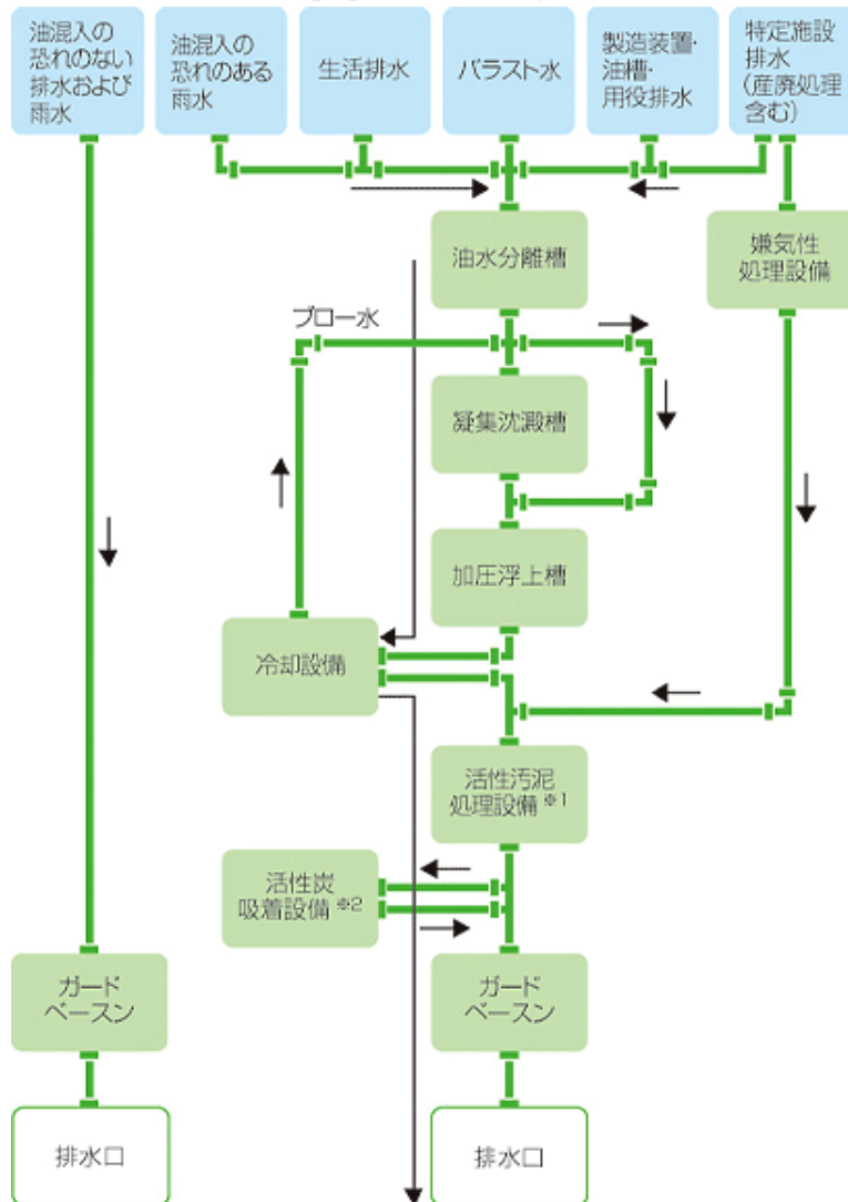
【図】汚水等の処理系統
