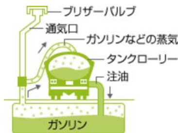
炭化水素ベーパーの回収
