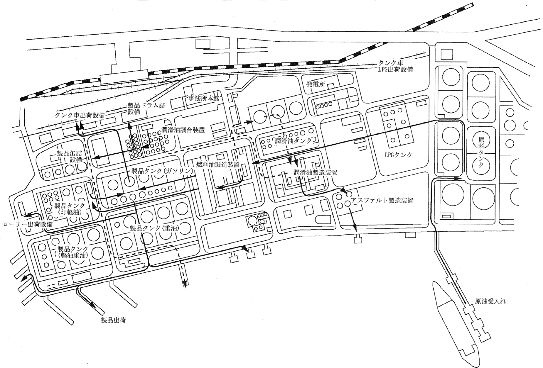
図 1-2-2-1 製油所の配置と油の流れ図の一例
