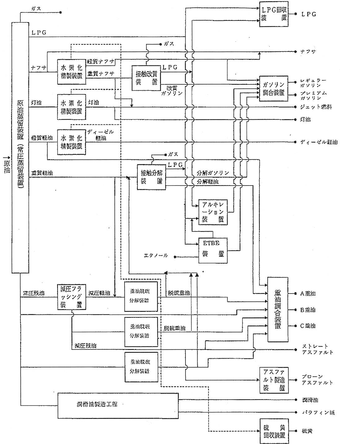
図 1-2-3-1 石油精製工程の一例
