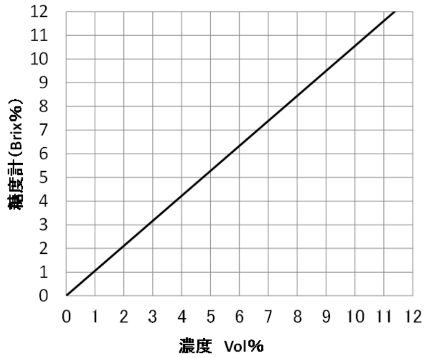
リライアソルス-PA(N)の濃度換算グラフ
