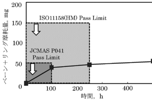
図5 V104C ベーパーポンプ試験による フードマシンハイドロ 32 の耐摩耗性評価結果
